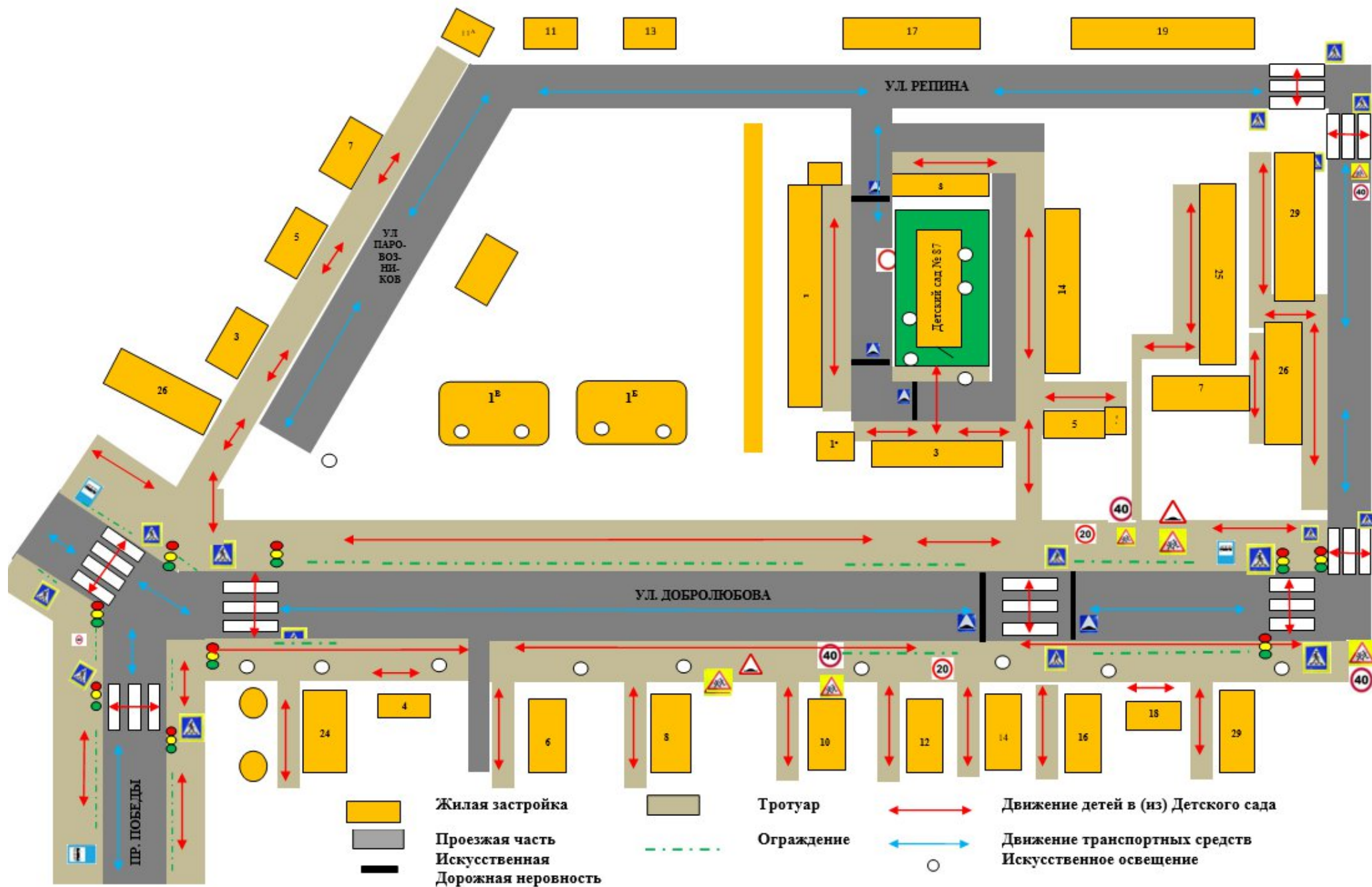
2. Схема организации дорожного движения в непосредственной близости от образовательного учреждения с размещением соответствующих технических средств организации дорожного движения, маршрутов движения детей и расположения парковочных мест
